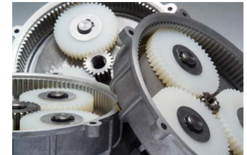
Langlebiges Planetengetriebe
